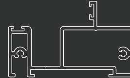
VISTO HEAD
